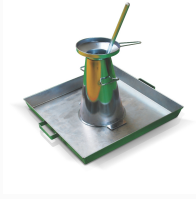
Slump-Çökme Deney Seti
